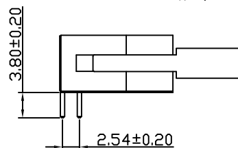
LONG LATCH (长勾)
