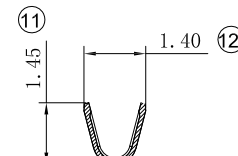
剖视图 B-B 比例 1:1
